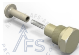
F074898 VÁLVULA DE RETENÇÃO (MOTOR HID. DA SERRA)
