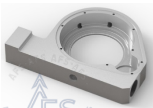
F073431 CARCAÇA (p/bujão M40) (SUPER CUT 100)
