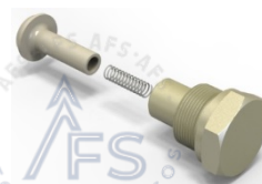
F074898 VÁLVULA DE RETENÇÃO (Motor Hid. do Sabre)
