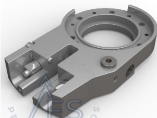
5240768 CONJ. SUPORTE DO SABRE (sem válvulas)
