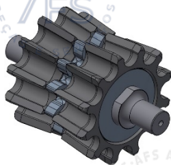
5250925 CONJ. ROLETE INTERMEDIÁRIO
