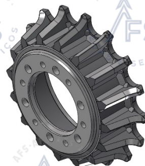
5334437-MOD (5251326) ROLO DE TRAÇÃO
