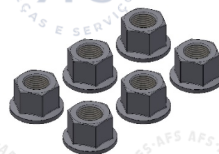
5079446 KIT - PORCAS M18 (6x) (FIX. DO ROLO NO MOTOR POCLAIN)
