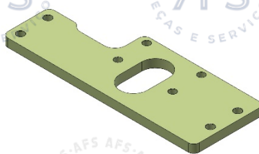
5233414 CHAPA P/ FIXAÇÃO DO COMANDO
