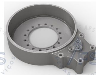
5090162 (5277208) CARÇAÇA
