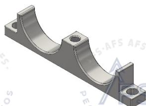
5280441 ABRAÇADEIRA INF. P/ ACUMULADOR
