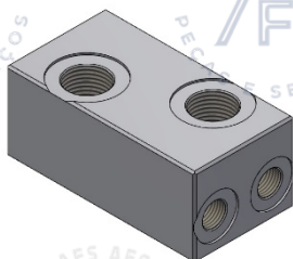
5280433 BLOCO
