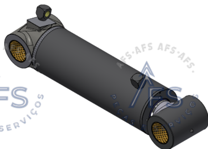
5279596 CILÍNDRIO HIDRÁULICO - ELEV.
