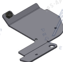
F657809 PROTEÇÃO
