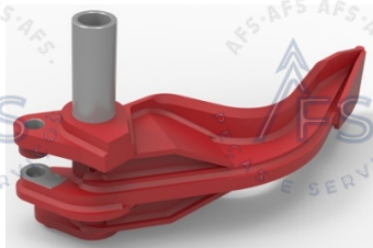
WA113858 (modelo soldado) FACA SUPERIOR ESQ. (p/622B)
