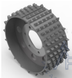
WA126313 ROLO DE TRAÇÃO (c/ Barras Dentadas)
