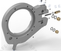
WA124901 CONJ. GRAMPO DO SABRE (p/ Unid.de Corte 3/4" c/ Tens.Automático)
