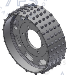
WA118478 ROLO DE TRACÇÃO (opcional c/ cravilhos)
