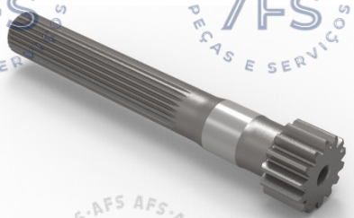
5236312 (L=440mm) EIXO - ENGRENAGEM SOL (Z=14) PLANETÁRIA - BOGIE - FW.895
