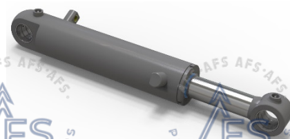
4691826 CILÍNDRO HID. DA GARRA G40HD (Padrão CRANAB)
