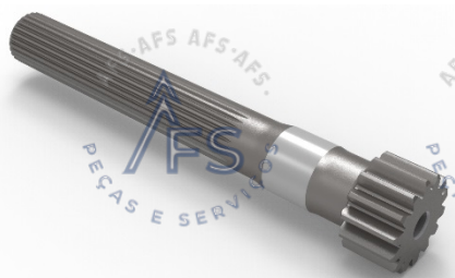
5236308 (L=462mm) EIXO - ENGRENAGEM SOL (Z=14) PLANETÁRIA - BOGIE - FW.895
