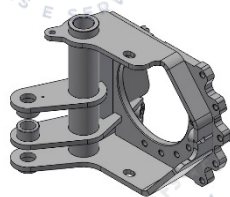
P33829 SUPOORTE DO MOTOR
