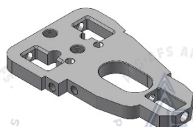
P15121 PLACA DE FIXAÇÃO
